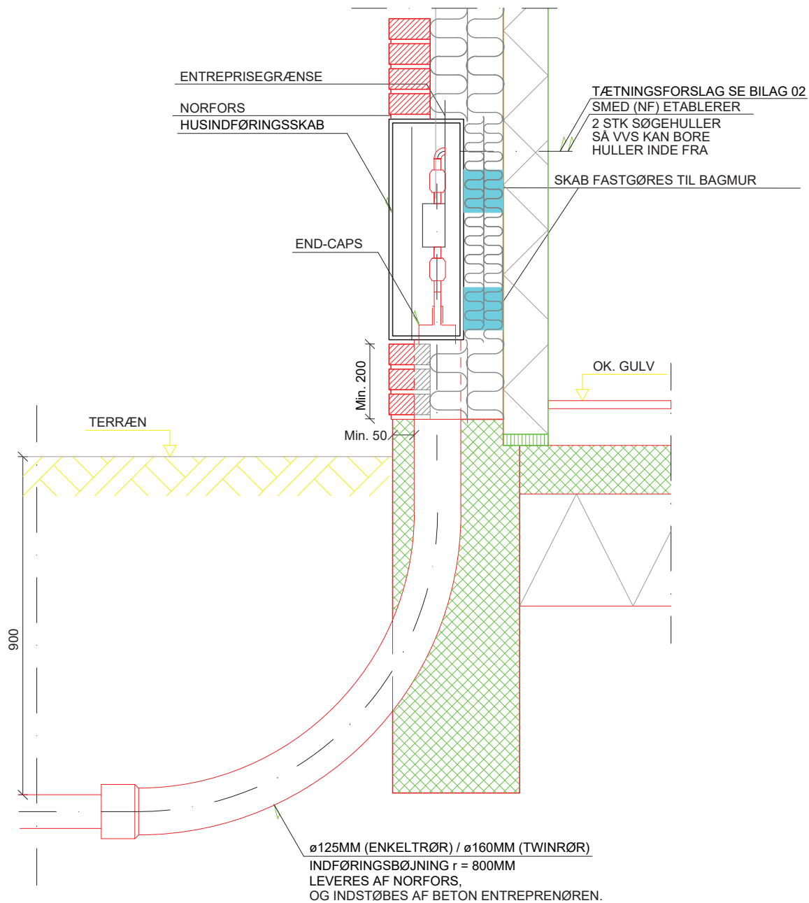
SNIT I HUSINDFØRING , 1:10
