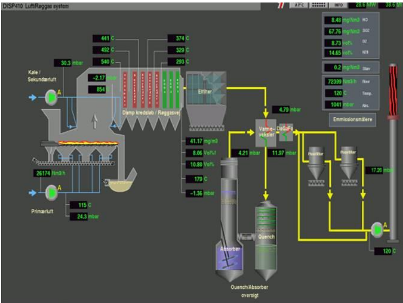
Procesdiagram for Ovnlíne 4
